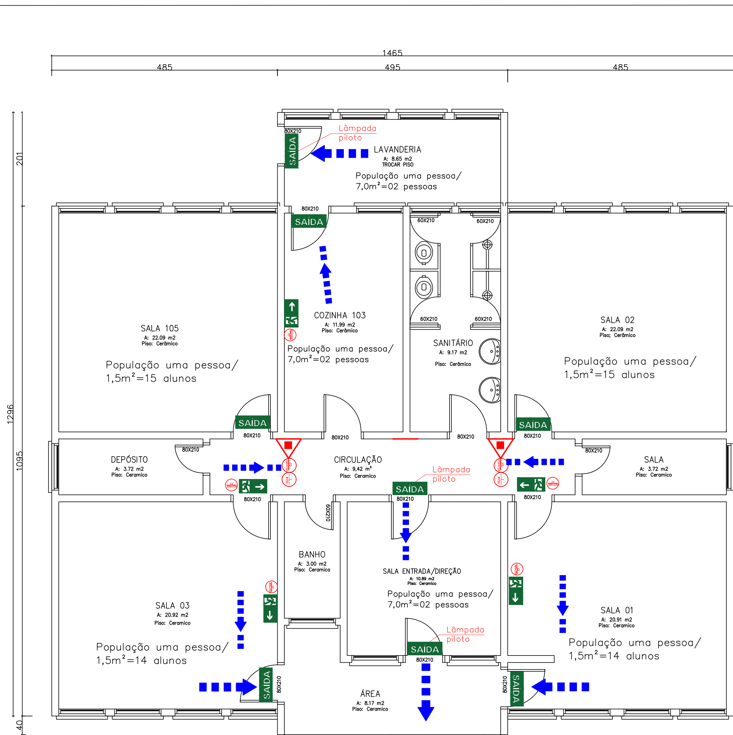
PLANTA BAIXA Escala 1/50 - A= 172,35m 2
